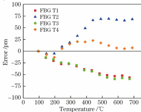
图 11 4 个光栅样品的普适性拟合函数误差
