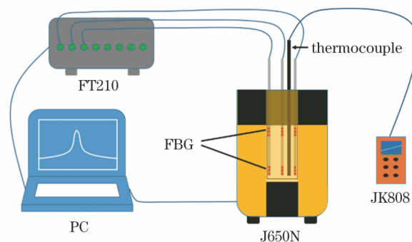
图5 FBG的退火与标定系统的装置图
