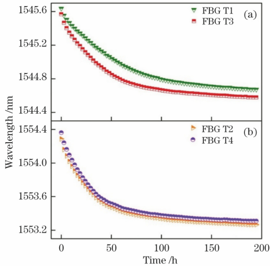
图 6 退火过程中 FBG 中心波长随时间的变化曲线。
