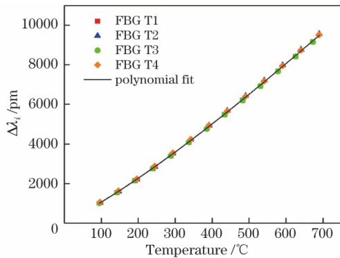
图 10 4 个光栅样品波长变化量与温度的拟合曲线
